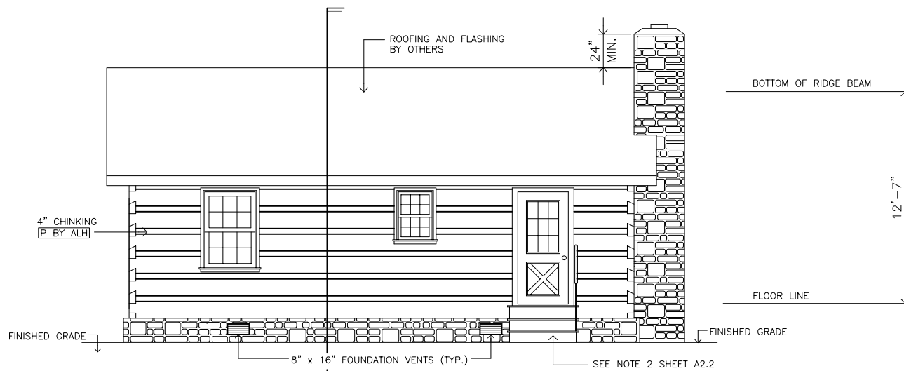
1 A3.2 HIWASSEE I REAR ELEVATION SCALE: 1/8" = 1'-0"
