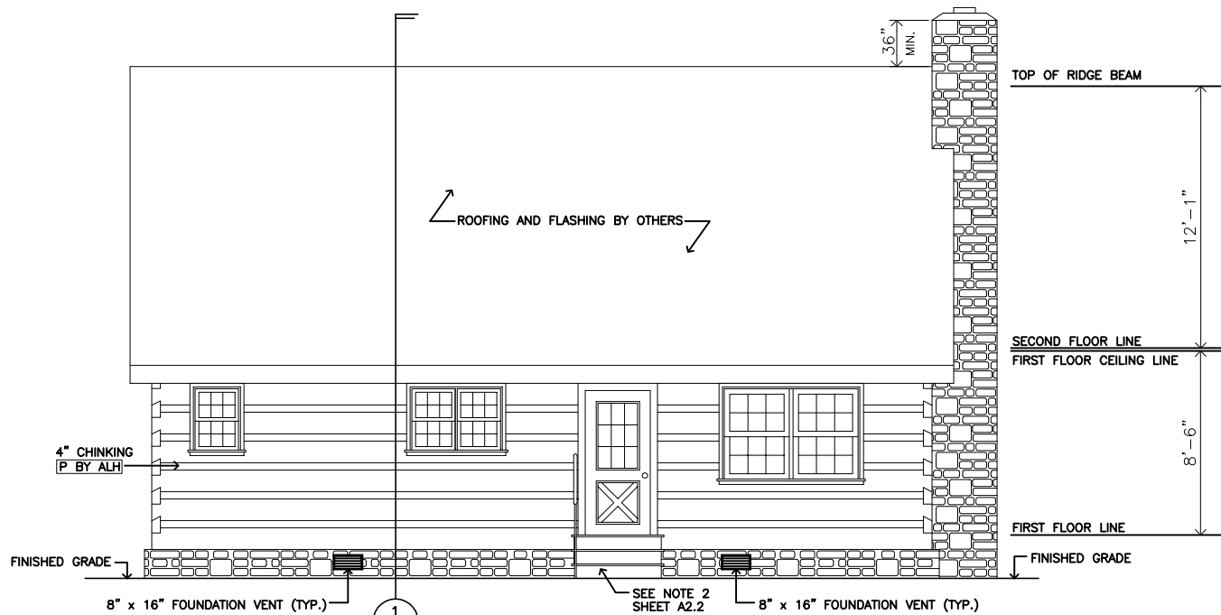
1 REAR ELEVATION A3.2 SCALE: 1/8" = 1'-0"
