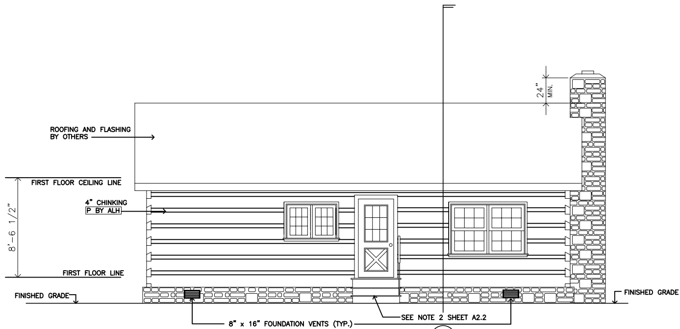
1 REAR ELEVATION A3.2 SCALE: 1/8" = 1'-0"
