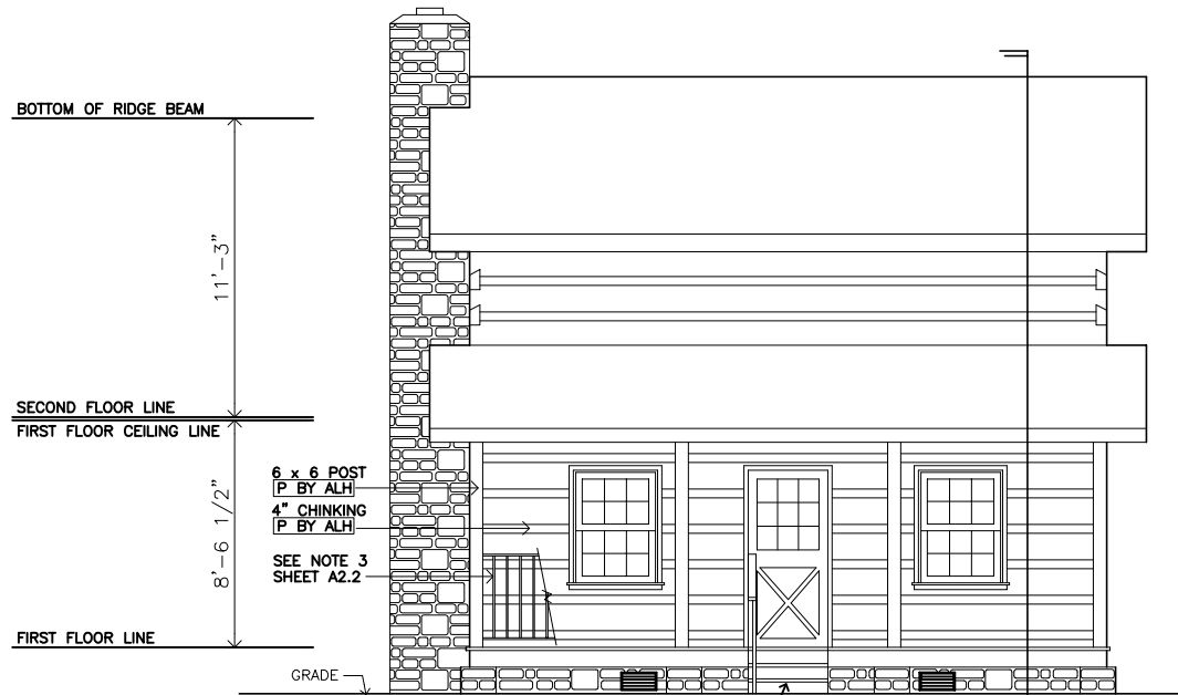
1/A3.1 FRONT ELEVATION SCALE: 1/8" = 1'-0"
