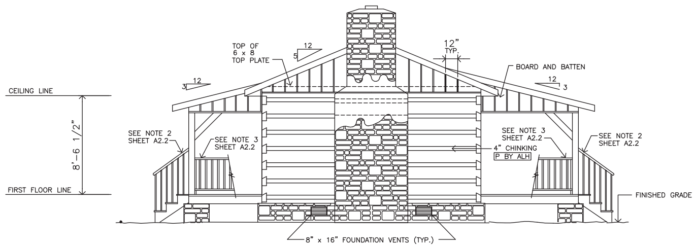
2 A3.2 LEFT ELEVATION SCALE: 1/8" = 1'-0"
